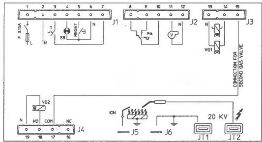
TYPE CM32
