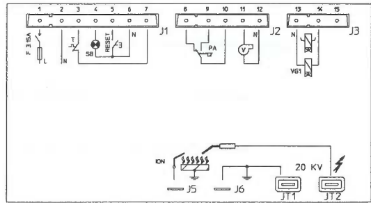
TYPE CM31
