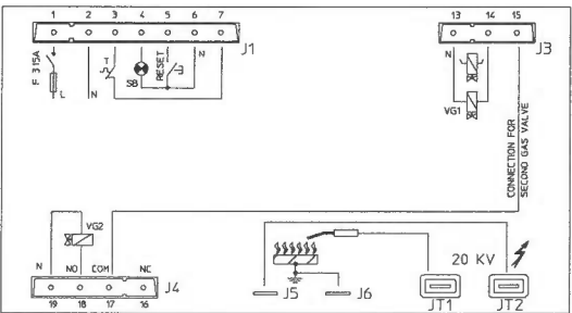
TYPE MM51
