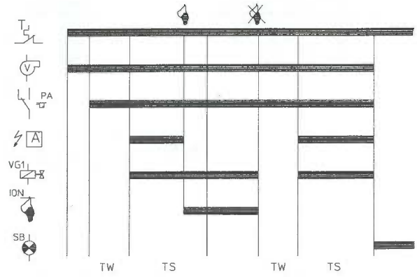
TYPE CM31
