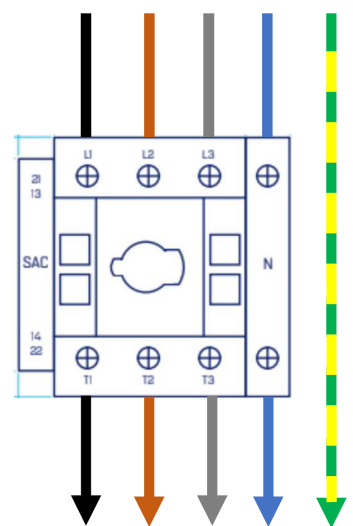
Branchement tétrapolaire - 4P Triphasé + neutre
